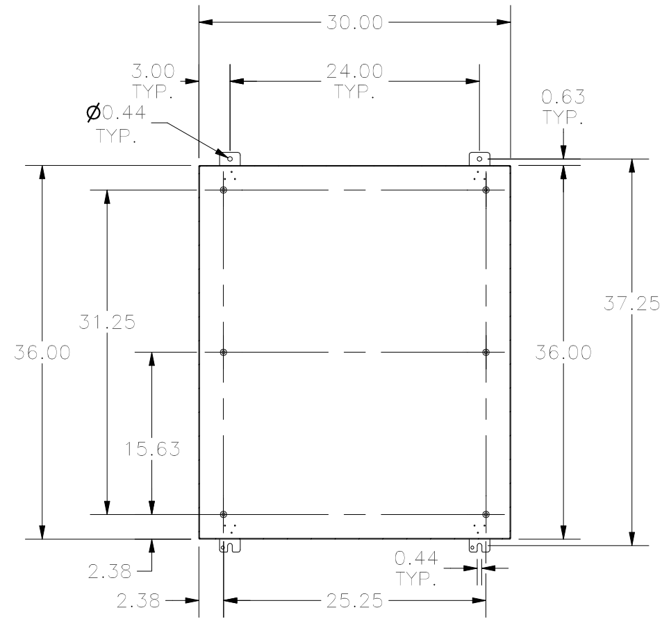
SECTION A-A
