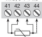
RTD, 3- / 4-fils
