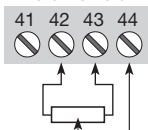
Potentiometer
