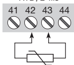
Résistance, 3- / 4-fils
