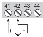
Transmetteur 2-fils
