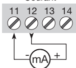
Courant
