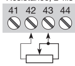
Résistance, 2-fils
