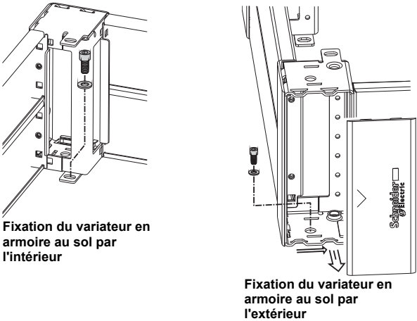
Figure 4 : Emplacement des trous de montage pour une fixation au sol
