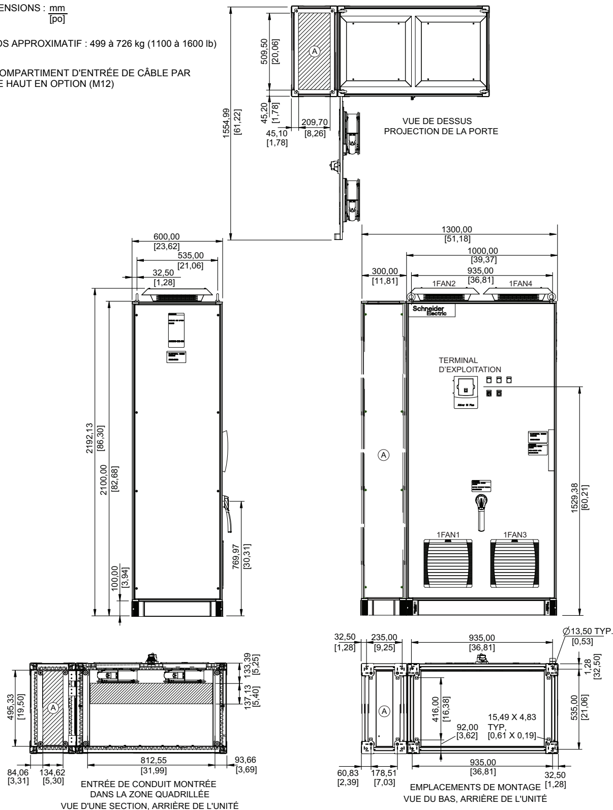
Figure 7 : Armoire châssis taille B : 350 à 500 HP CV et 250–450 HP CC à 460 V, 250 à 450 HP CV et 200 à 350 HP CC à 575 V, sectionneur à fusible pour 460 V et 575 V
