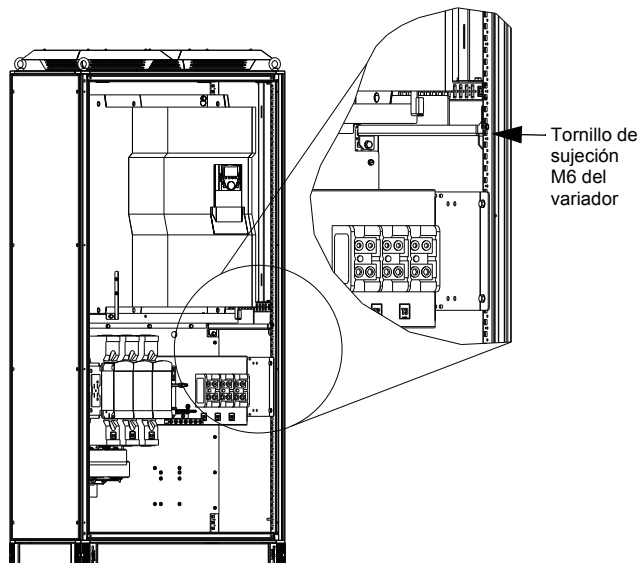
Figure 15: Desmontaje del ensamble del variador
