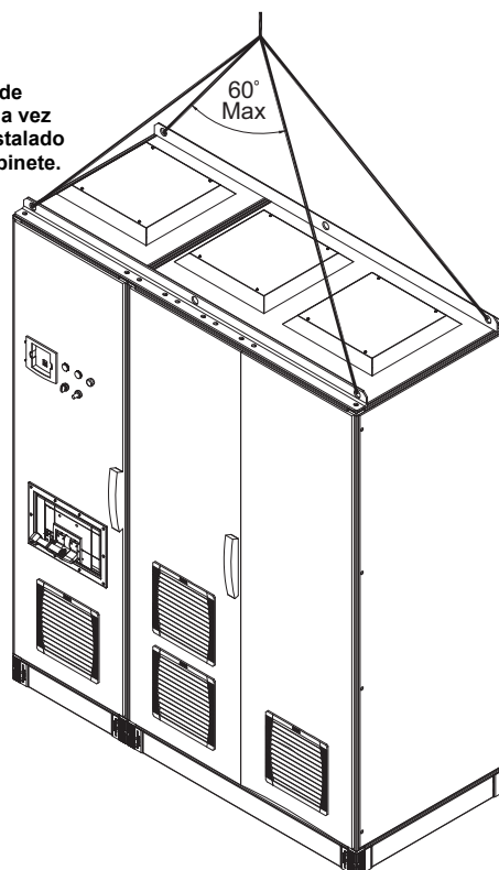
Figura 3: Levantamiento con equipo elevador (marco C)
