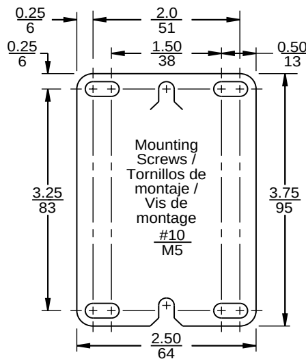
Figure / Figura / Figure 3 Contactor Mounting Dimensions Dimensiones de montaje del contactor Dimensions de montage du contacteur
